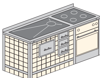
Kombiniran štedilnik na trdo gorivo s pečico s pripravo za vgradno ploščo in pečico
